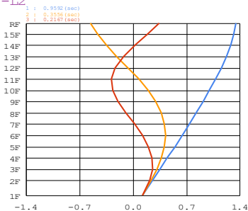
モード形状 (刺激関数)
