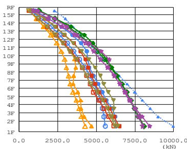
最大応答層せん断力 (kN)
