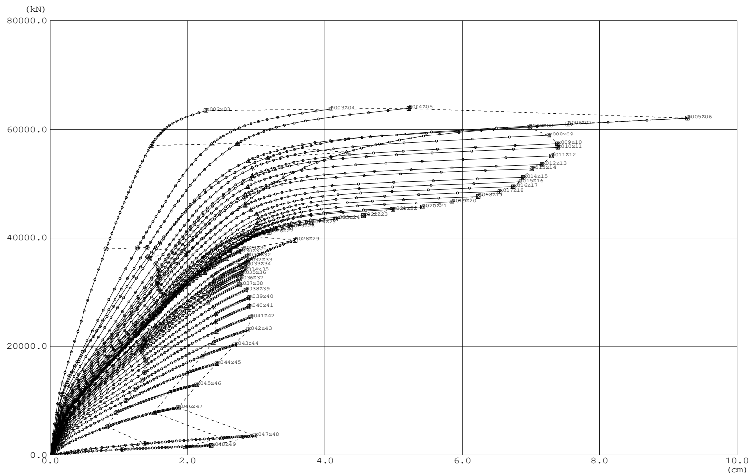
層せん断力－層間変位図（+X方向）
