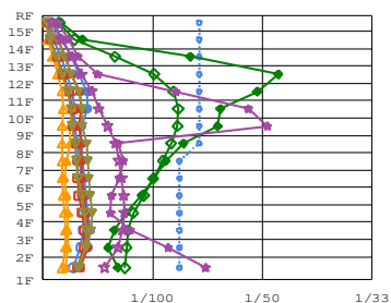
最大応答層間変形角 (Rad.)
