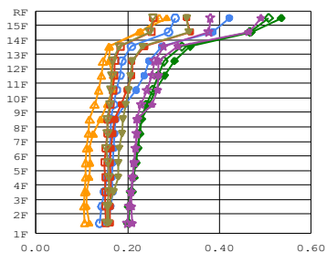
最大応答層せん断力係数
