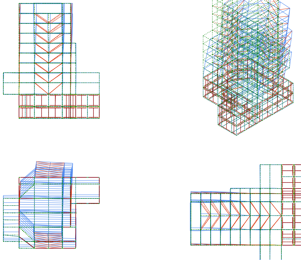
三面固有モードベクトル図 ( )
