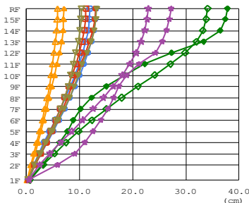
最大応答変位 (cm)
